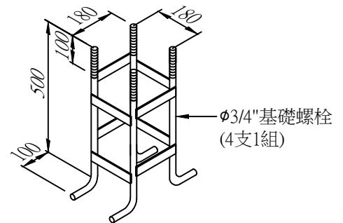
基礎螺絲詳圖
