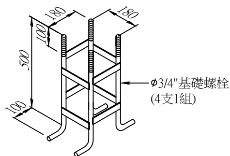
基礎螺絲詳圖
