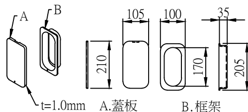
補強型維修孔詳圖
